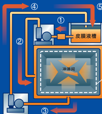
地下坑型
